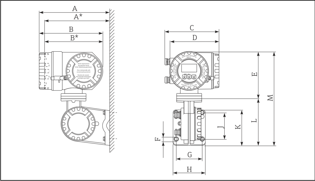
分体式变送器的接线盒 (H2G / 1 区 )
